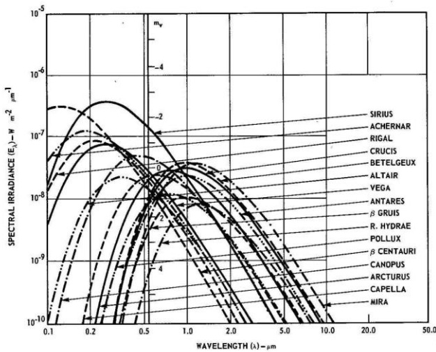
Rys. 2. Rozkład spektralny promieniowania najjaśniejszych gwiazd, na zewnątrz atmosfery, jako dowód, że ich sumaryczna energia jest o dziewięć rzędów niższa i może nie być brana pod uwagę, a Słońce jest podstawowym źródłem energii docierającej do Ziemi.
