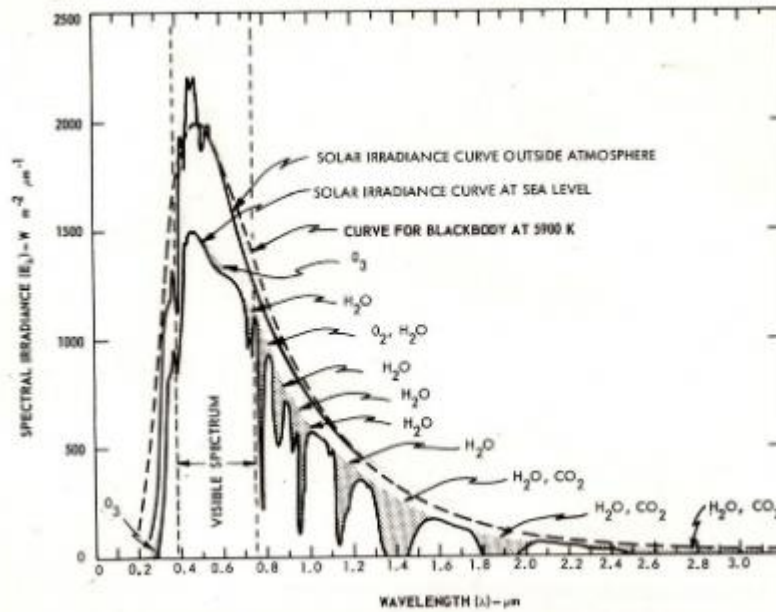
Rys. 1. Rozkład spektralny promieniowania słonecznego, z zaznaczonymi pasmami absorpcji składników gazowych atmosfery. ( RCA Corp. (1984): Electro - Optics Handbook, Technical Series EOH -11, Printed in USA 74/8} Przedstawiony jest tu wykres energii na zewnątrz atmosfery i wykres energii docierającej do Ziemi, mierzony na poziomie morza.
