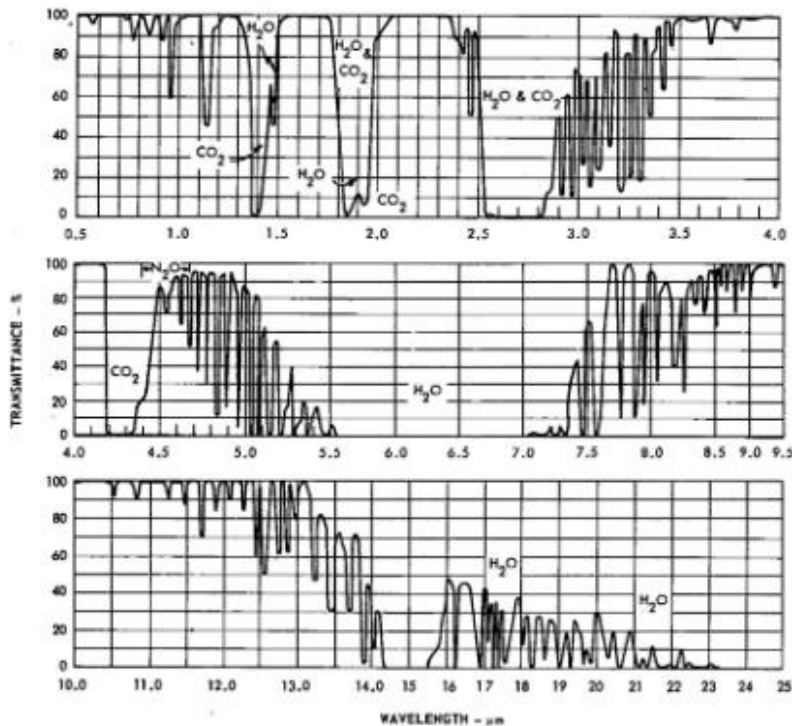
Rys. 4. Transmisja atmosfery.
