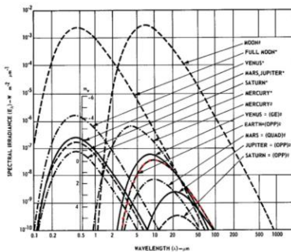
Rys. 3. Wyliczony rozkład spektralny promieniowania planet. (Rys.2 i3 wg.: Ramsey, R.C. "Spectral Irradiance from Stars and Planets, above the Atmosphere from 0,1 to 100,0 Microns", APPLIED OPTICS, Vol. 1, No 4 July1962)
